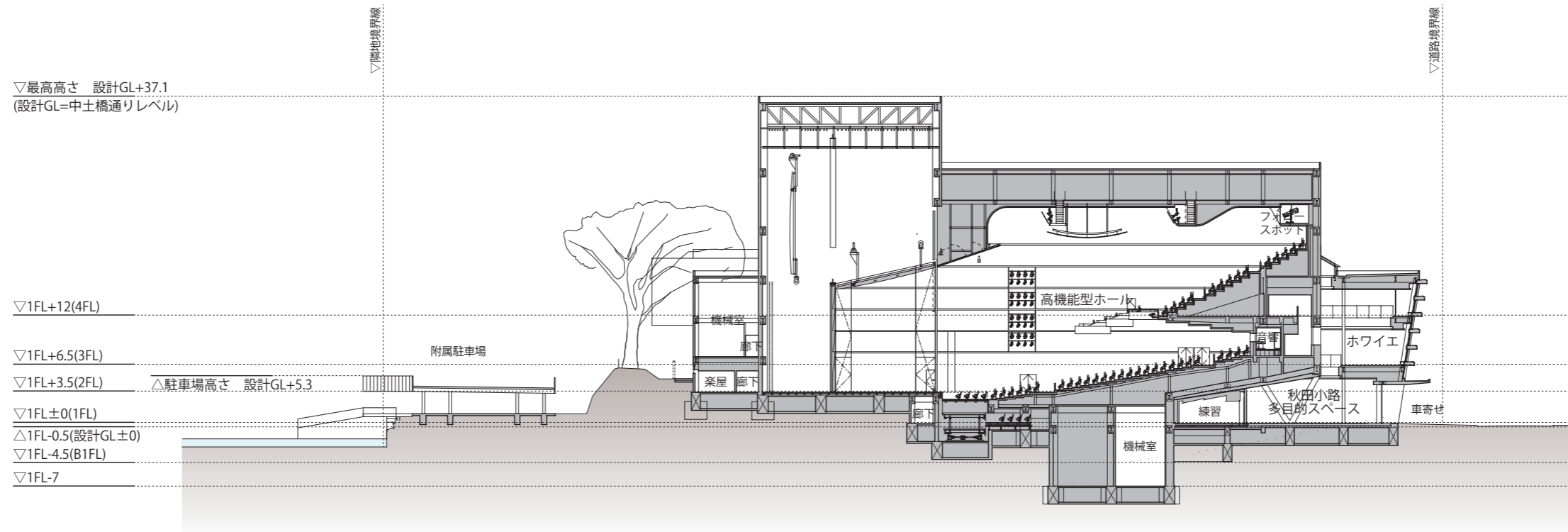
高機能型ホール断面
