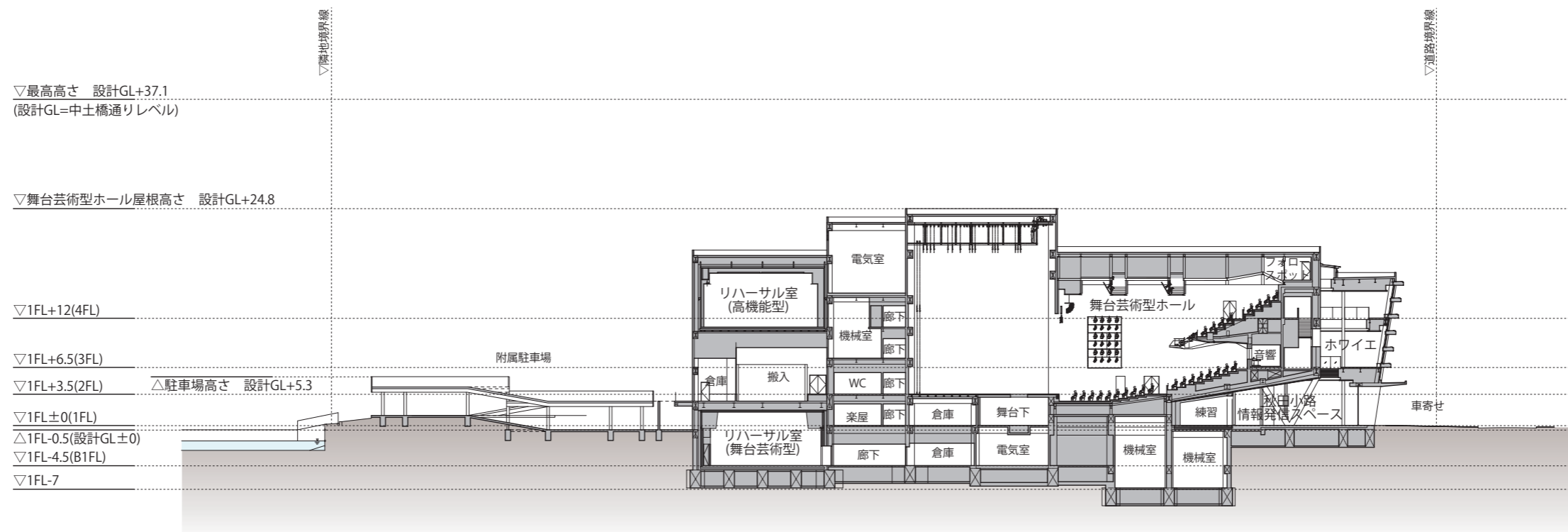
舞台芸術型ホール断面
